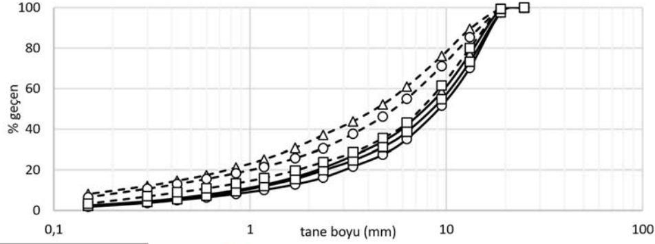
Şekil 1. Tane boyu dağılımları
